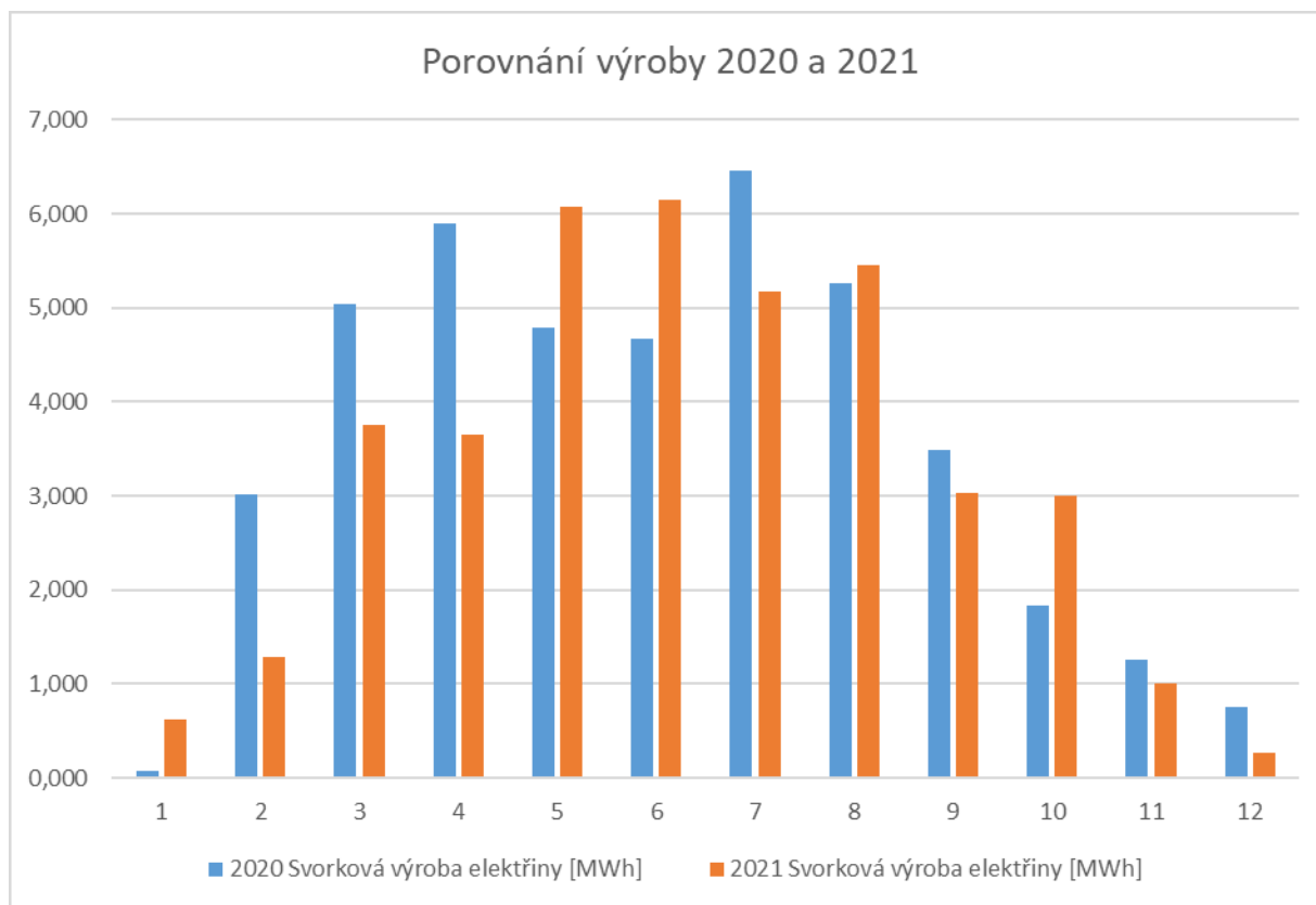
Svorková výroba elektřiny v roce 2020 a 2021
